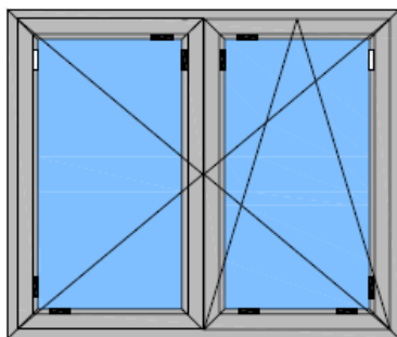
Fereastră în două canate mobile
